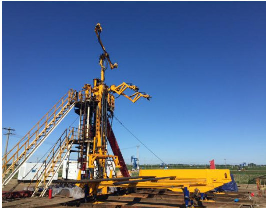
石油井口起下管机械手（一代）
