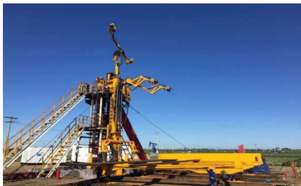
石油井口起下管机械手（一代）
